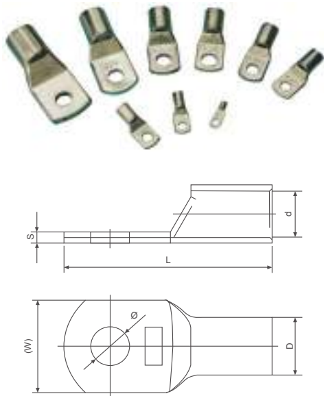
Медные клеммы SC(JGK)
