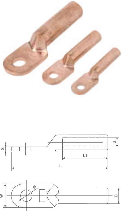
Медные соединительные клеммы DT
