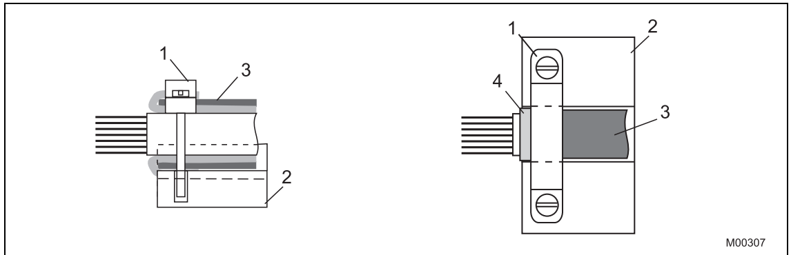
Рис. 13: Монтаж экрана кабеля
