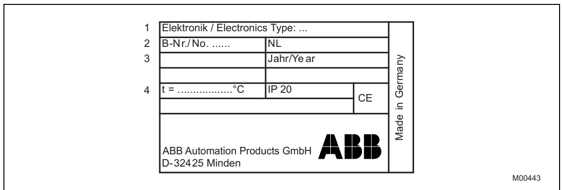
Рис. 4: Фирменная табличка на кожухе электронного блока, аппаратная часть
