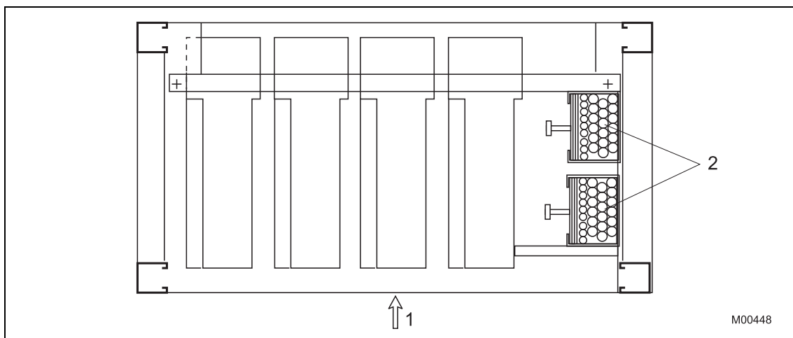
Рис. 22: проводка кабелей и монтаж электронных блоков внутри стойки (вид сверху)
