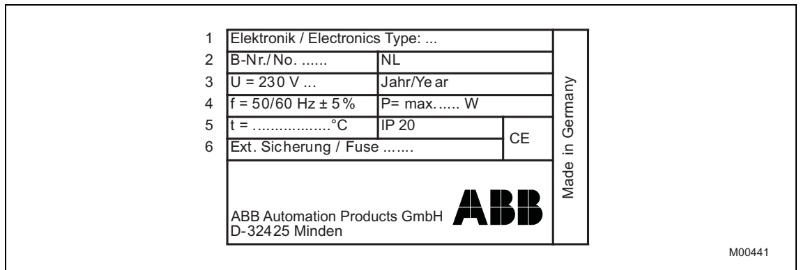
Рис. 3: Фирменная табличка на нижней части электронного блока
