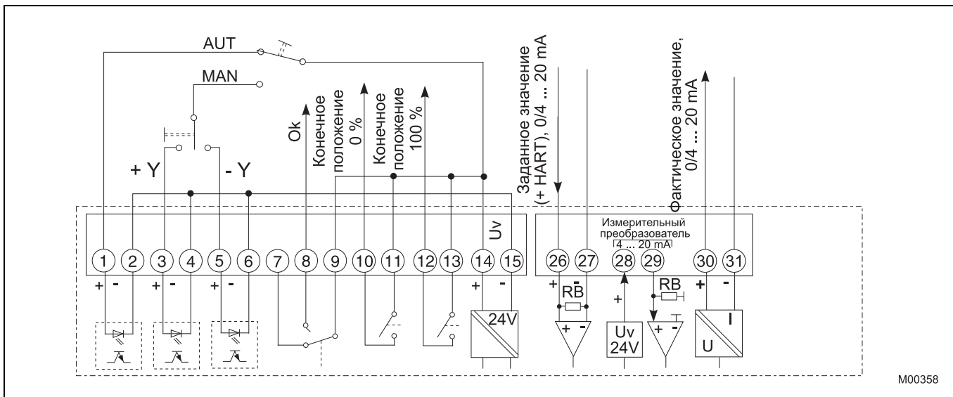
Рис. 17: Вариант разводки для стандартного назначения выводов при конфигурации по умолчанию
