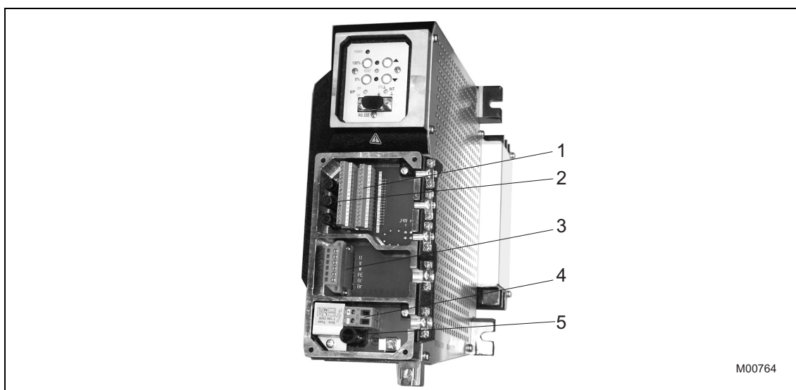
Рис. 8: Отсек подключения
