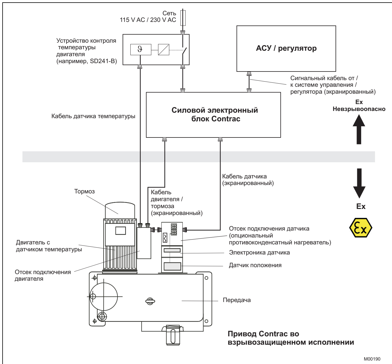
Рис. 6: Концепция взрывозащиты
