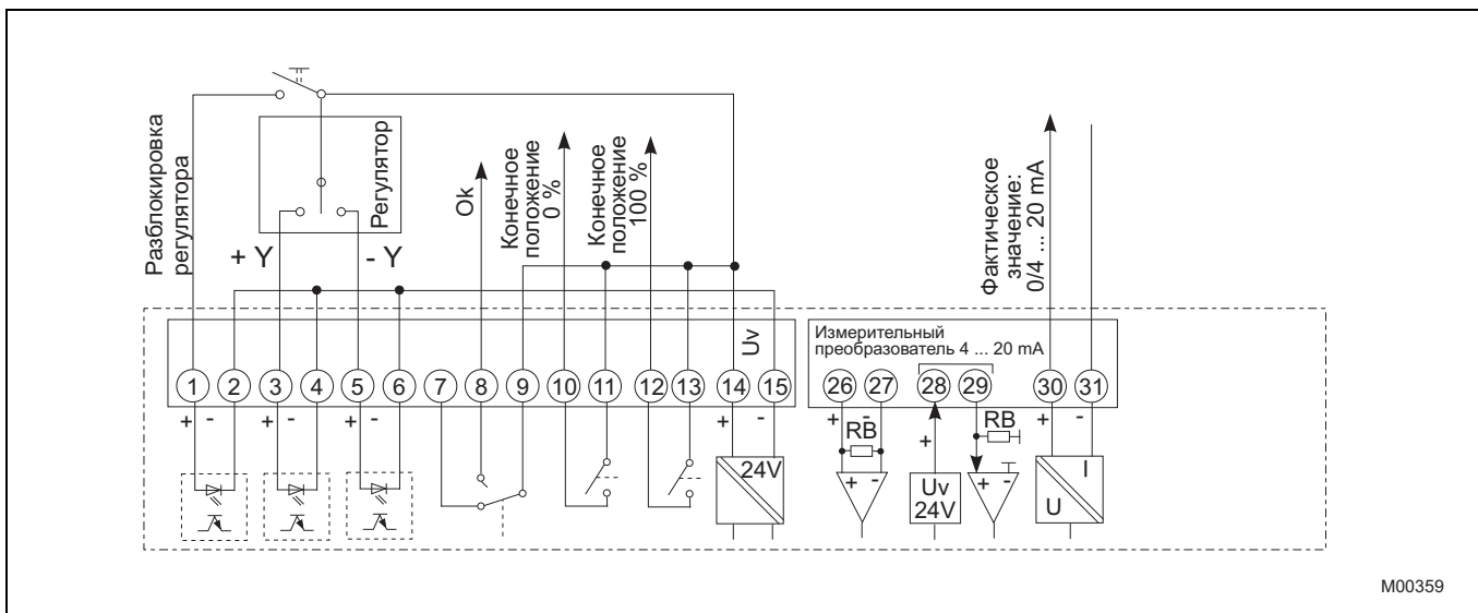
Рис. 18: Вариант разводки для «Работы по сигналу ступенчатого регулятора».
