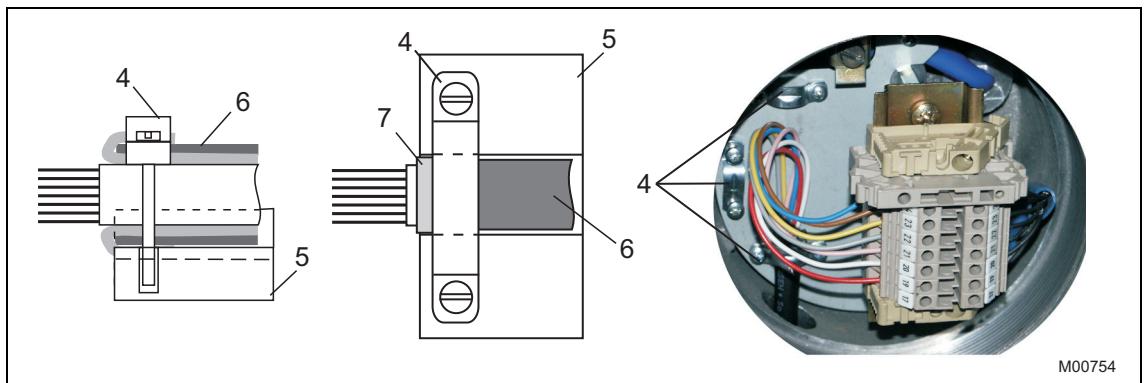
Рис. 12: Монтаж экрана кабеля
