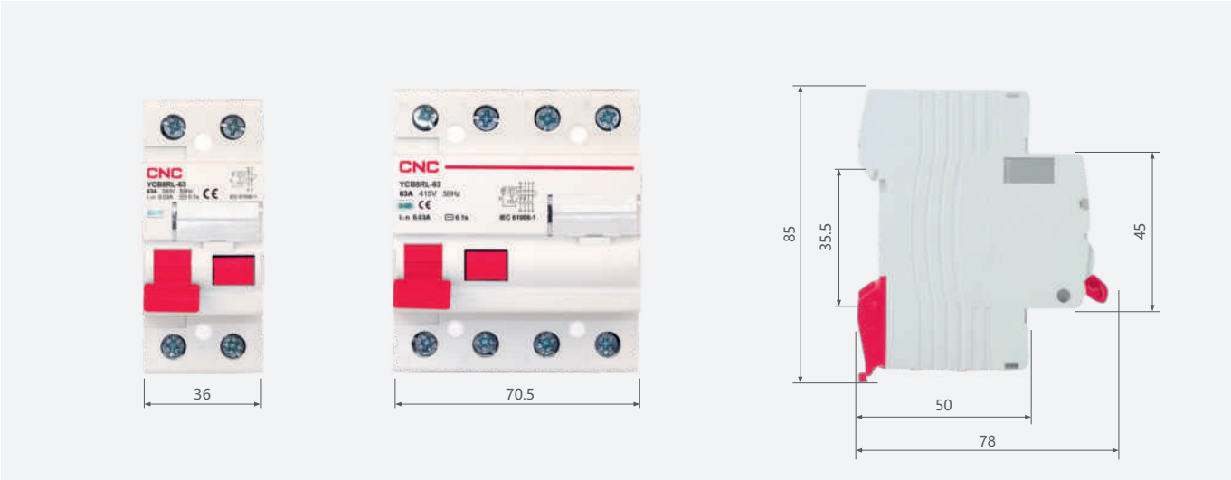
Габаритные и монтажные размеры (мм)
