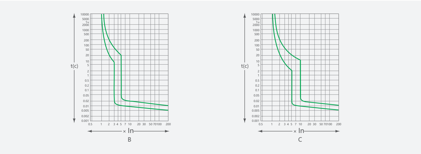
Времятоковые характеристики:
