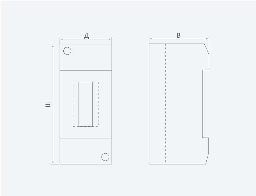
Габаритные и монтажные размеры (мм)
