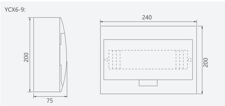
Габаритные и монтажные размеры (мм)
