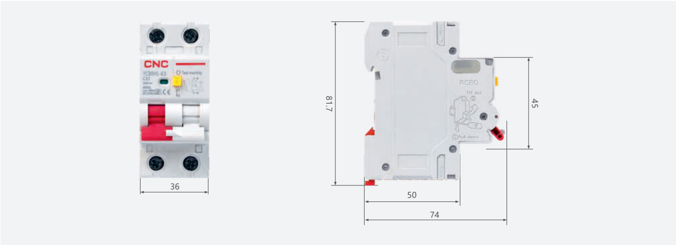
Габаритные и монтажные размеры (мм)
