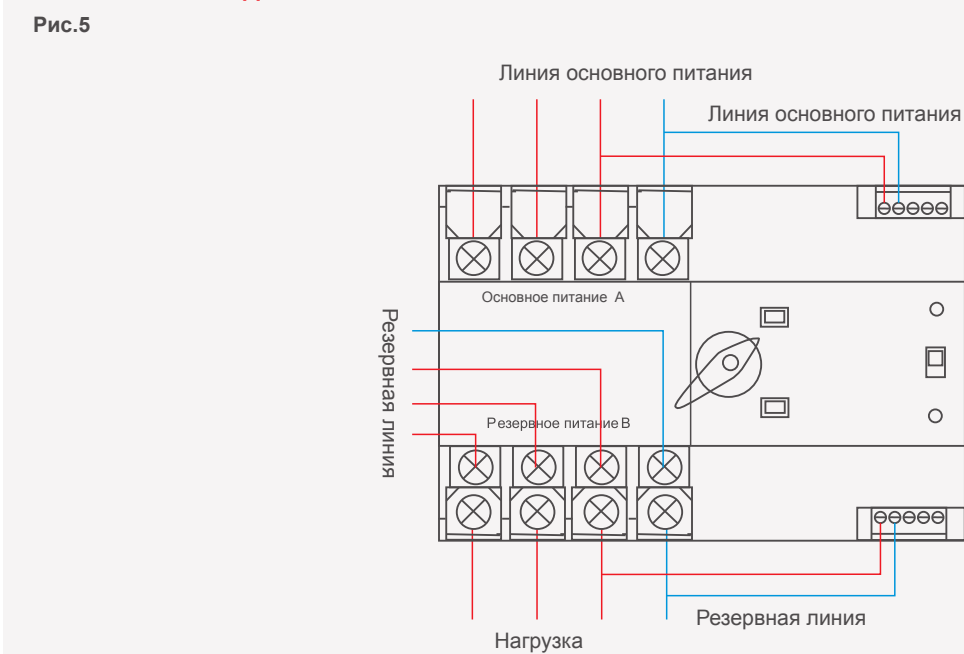
100/4P с хема подключения YCQ4E
