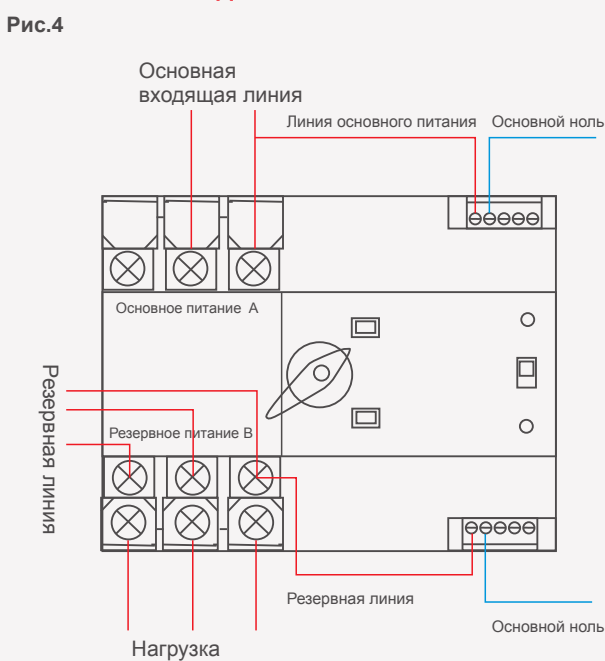
100/3P с хема подключения YCQ4E
