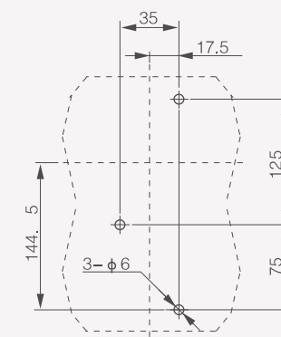
ЗР: монтаж на панель
