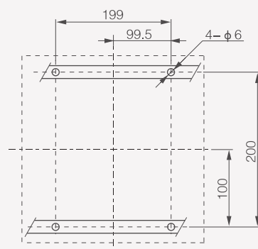
ЗР: монтаж на направляющие
