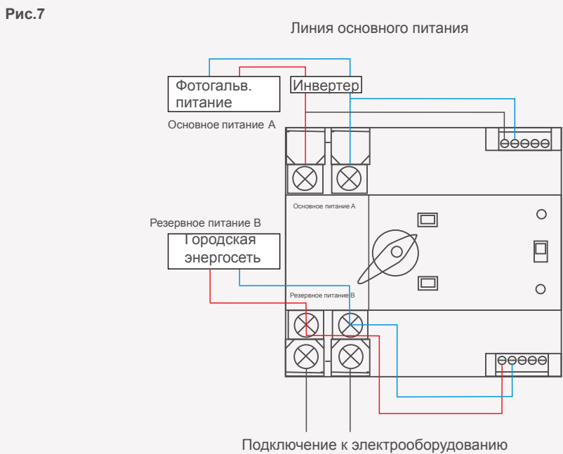
Специальный режим подключения фотогальванического инвертора YCQ4E
