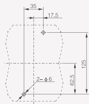
ЗР: монтаж на панели
