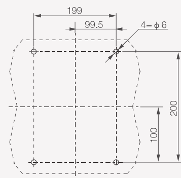
3Р: монтаж на панель
