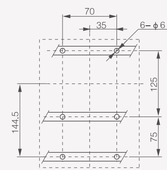
4Р: монтаж на направляющие
