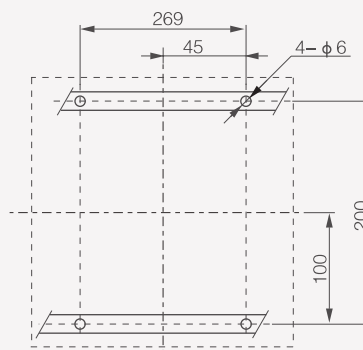
4Р: монтаж на направляющие
