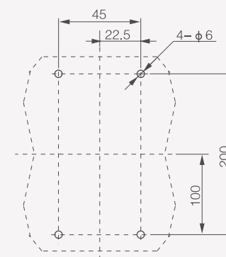
ЗР: монтаж на панели
