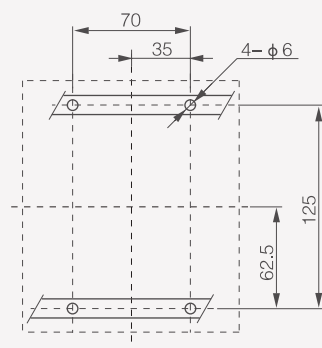
4Р : монтаж на направляющие
