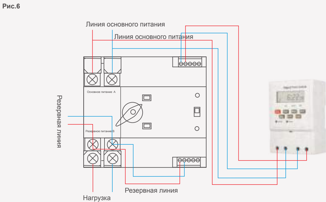
Режим переключения по времени YCQ4E
