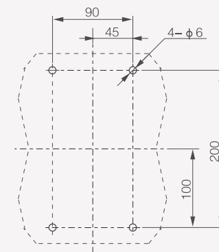
4Р: монтаж на панели
