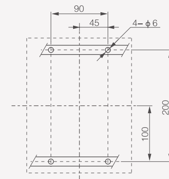
4Р: монтаж на направляющие
