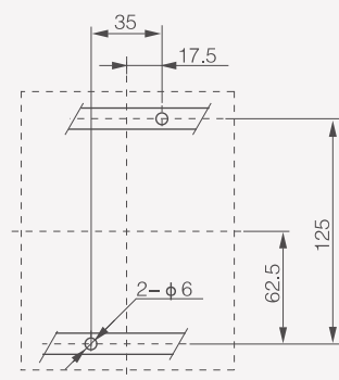
ЗР : монтаж на направляющие
