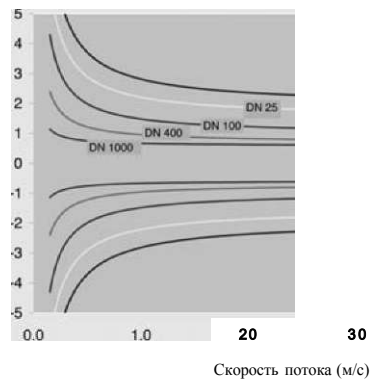
Типичная погрешность расходомеров Clamp-on для различных размеров труб
