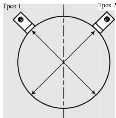
Пример установки с двойным лучом (Dual Beam)
