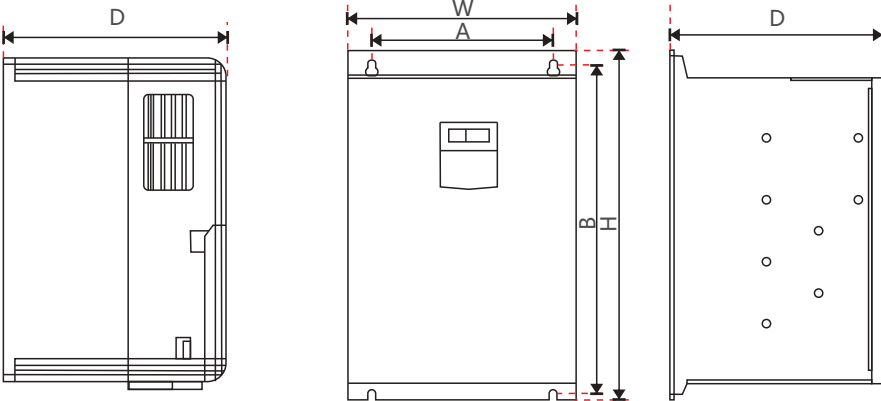
Рисунок А-1. Габаритные размеры для моделей мощностью до 7,5 кВт (380 В)
