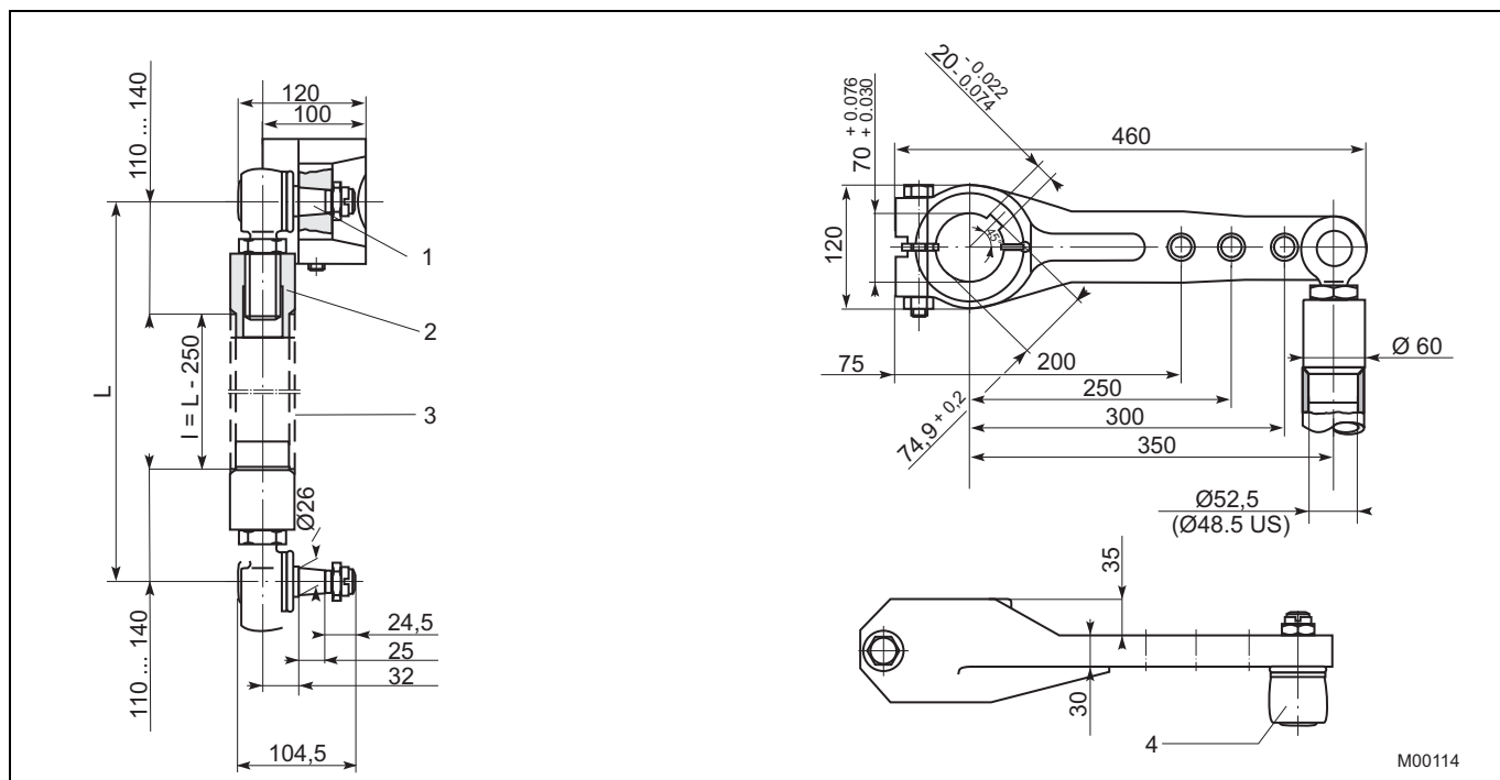
Рис. 9: габариты в мм
