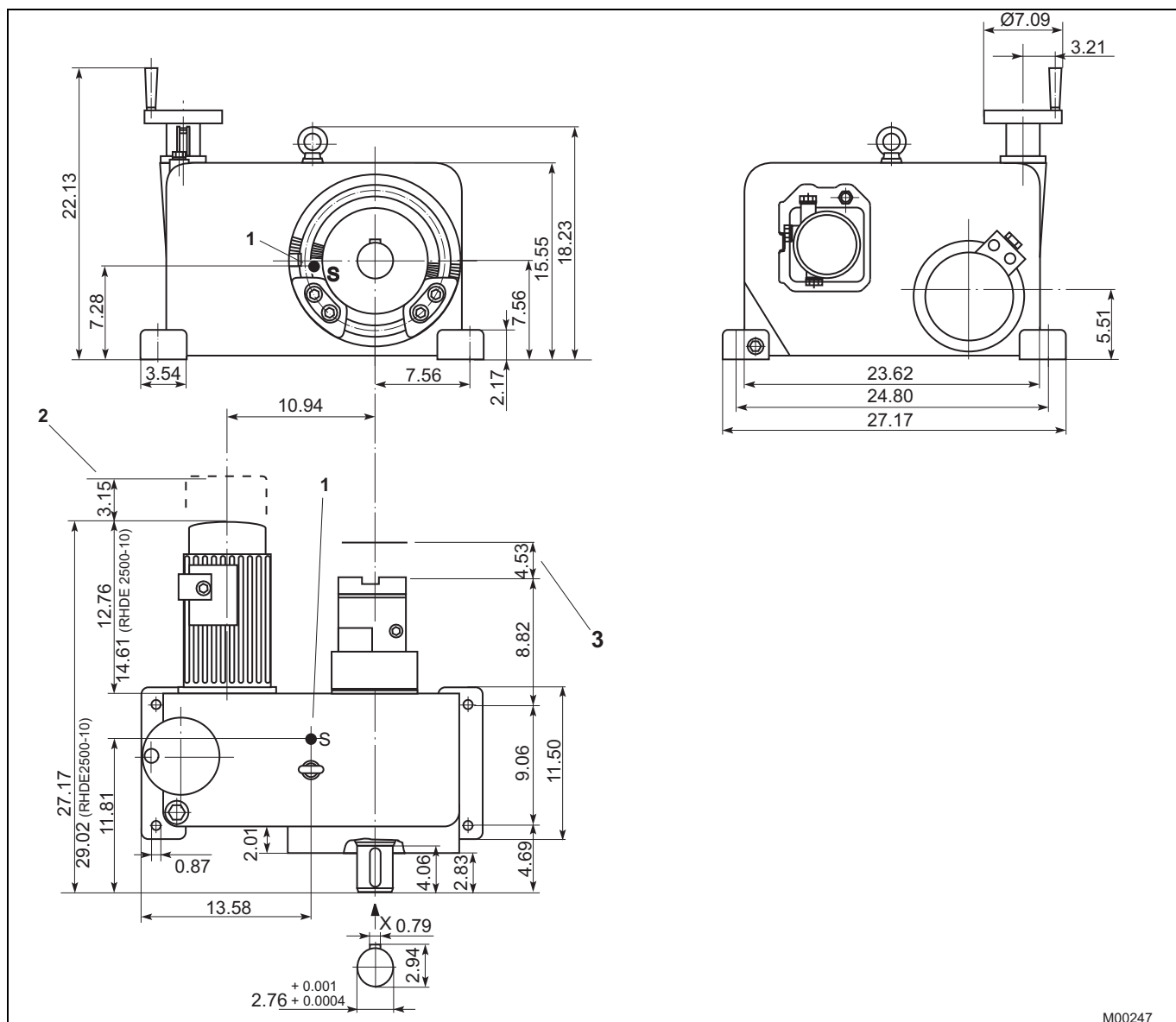
Рис. 8: габариты в дюймах
