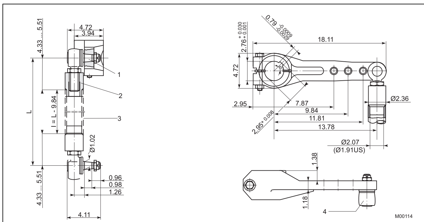
Рис. 10: габариты в дюймах
