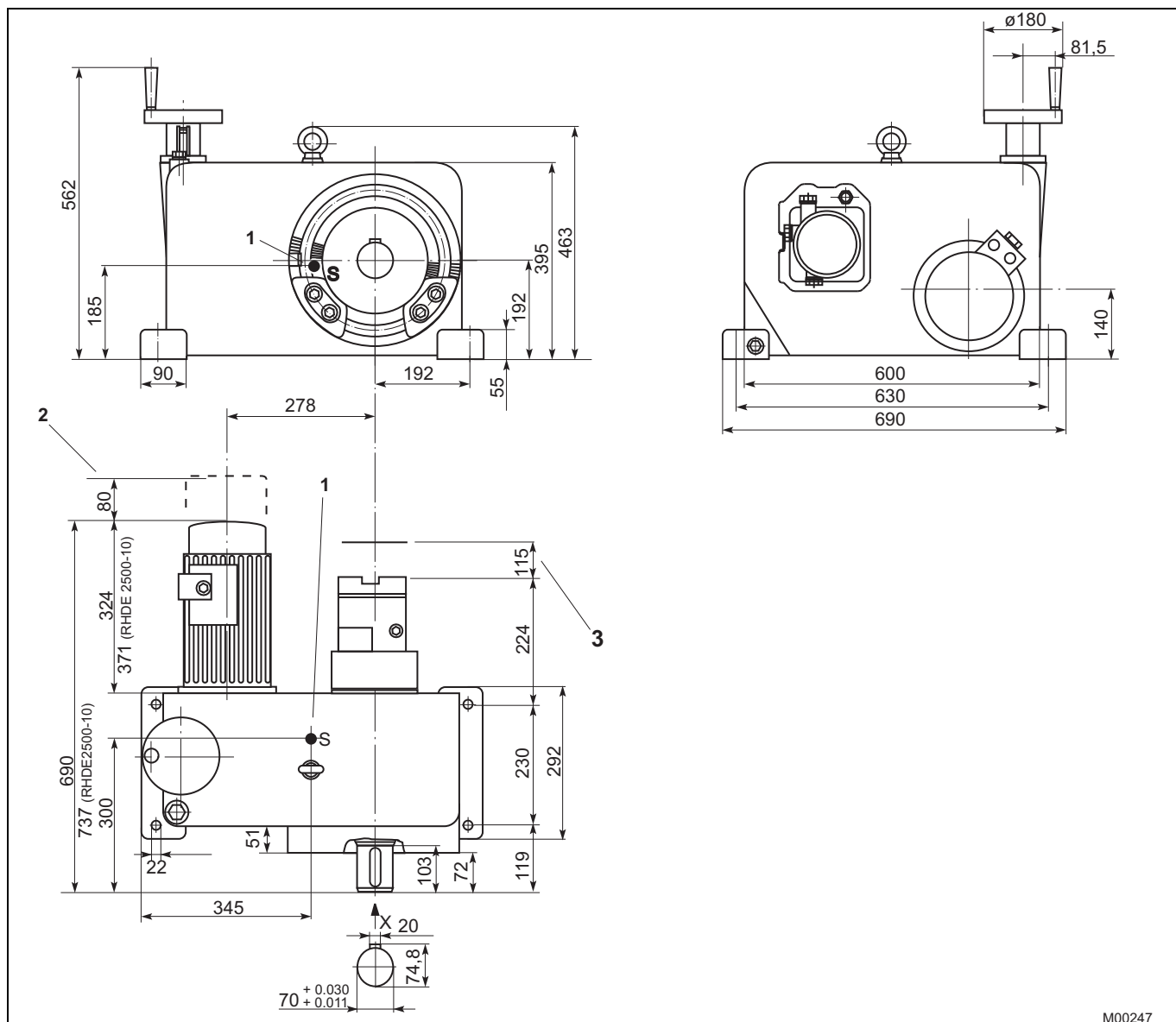
Рис. 7: габариты в мм
