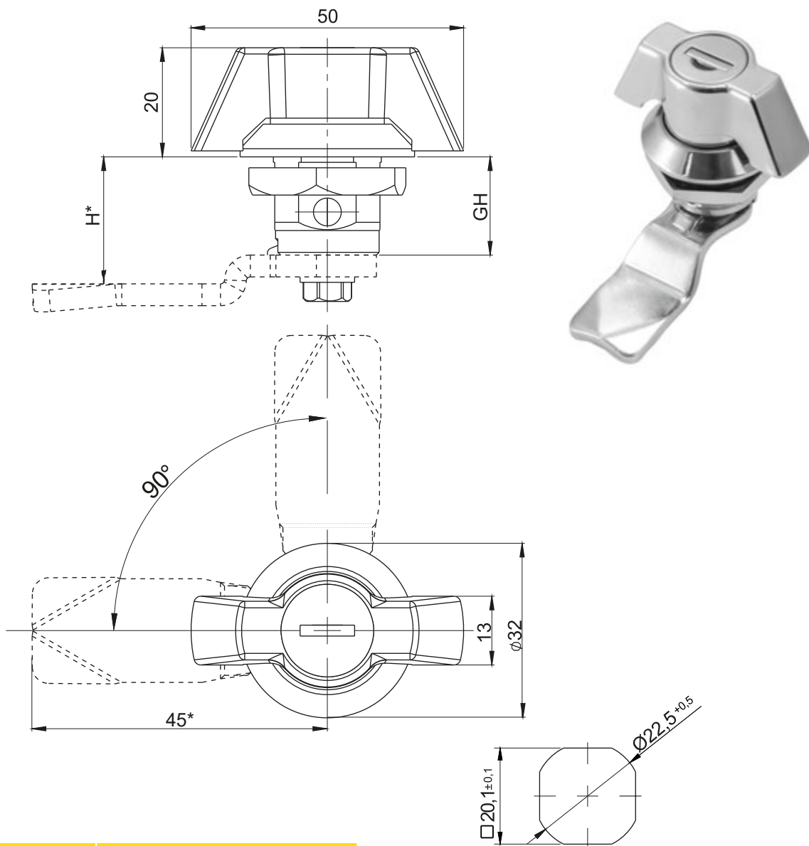
Монтажное отверстие
