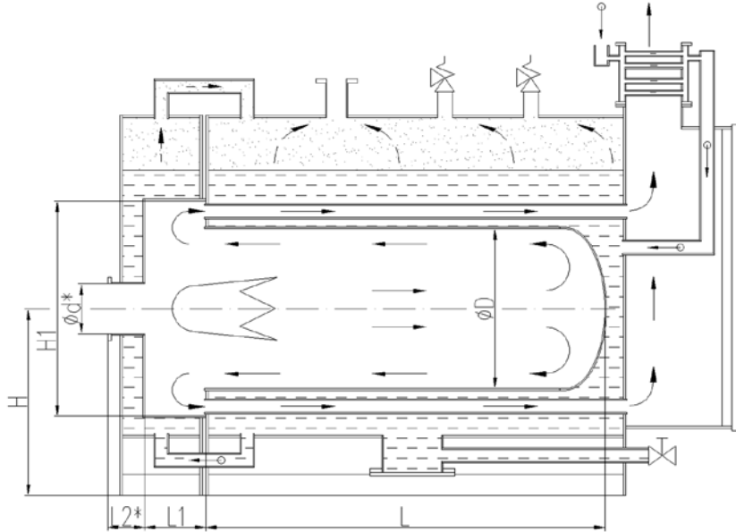
Рисунок 1– Технологическая схема КП-0,3-КП-2,0; КП-3,0-КП-10
