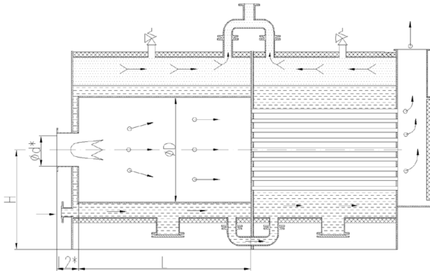
Рисунок 2– Технологическая схема КП-2,5
