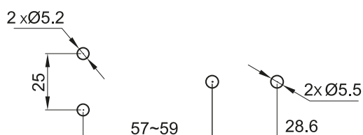
Монтажное отверстие
