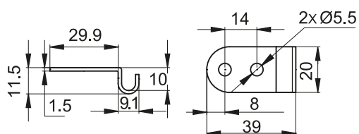
Монтажное отверстие
