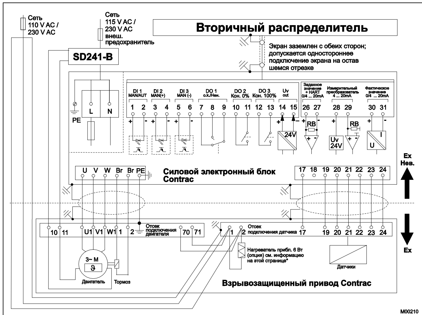
Рис. 3: электрическое подключение: взрывозащищенный привод аналоговый / двоичный
