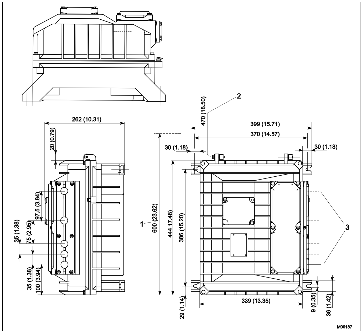
Рис. 5: габариты в мм (inch)
