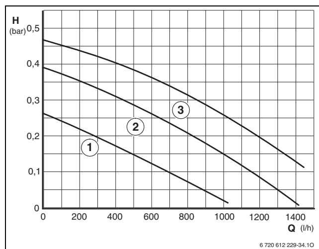
Рис 32 Характеристическая кривая насоса на Logamax U052-24/28K
