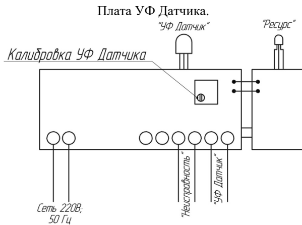
Рис.1 Плата УФ Датчика
