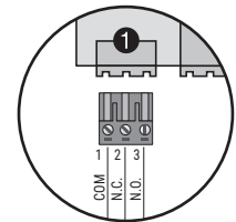
Relais Bedingung „Kein Alarm“
