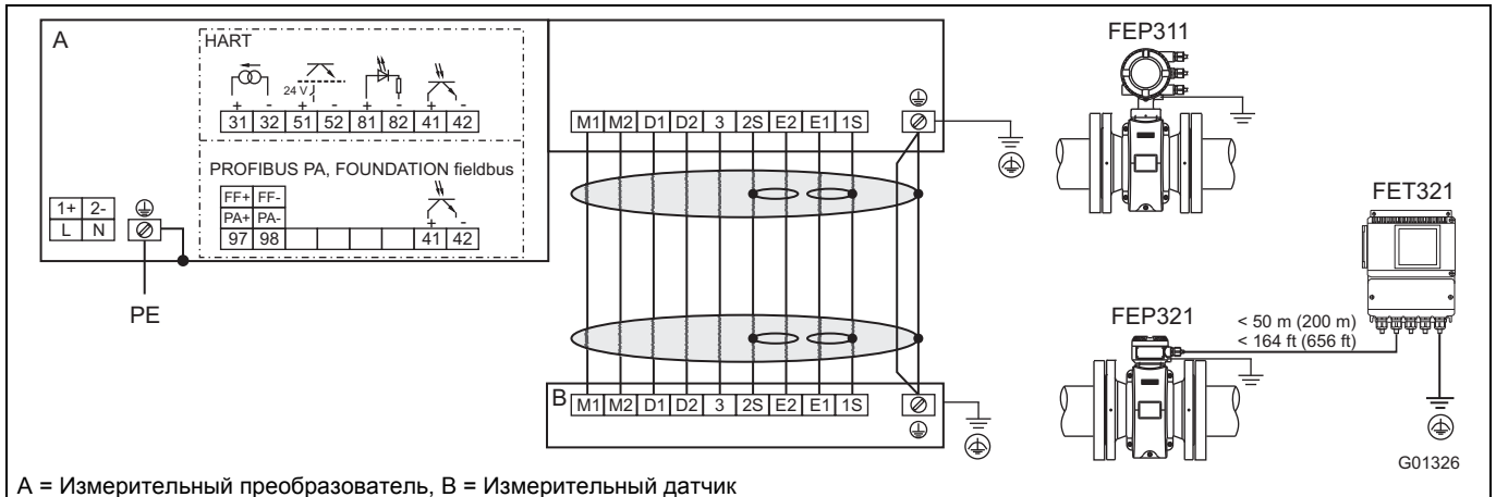
Рис. 12: Протоколы HART, PROFIBUS PA и FOUNDATION fieldbus
