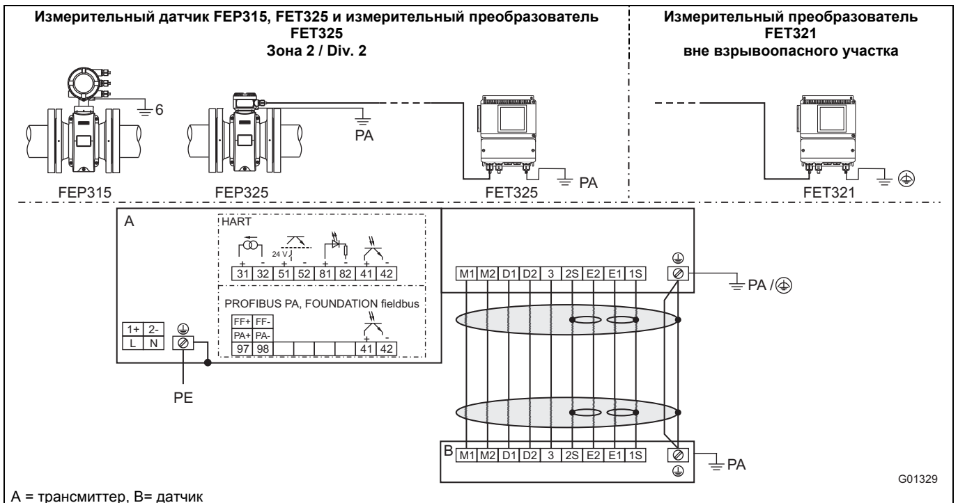
Рис. 26: Протоколы HART, PROFIBUS PA и FOUNDATION fieldbus
